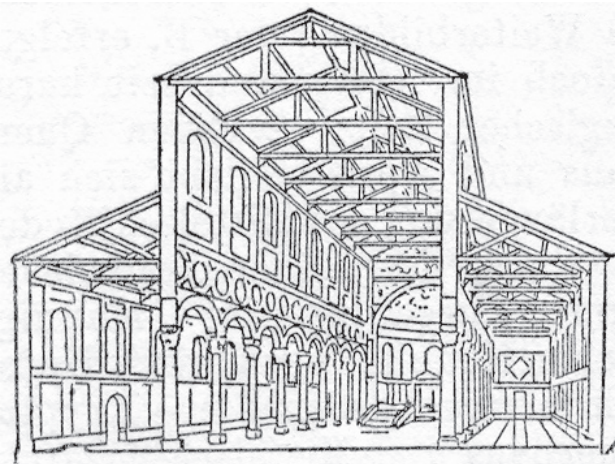
A bazilikális felépítés keresztmetszeti ábrázolásban
