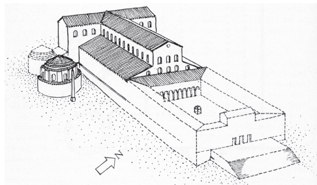
Az ősi Szent Péter-templom Rómában – a ma is álló templom reneszánsz építészei által a lebontás előtt készített felmérési rajzok szerint
