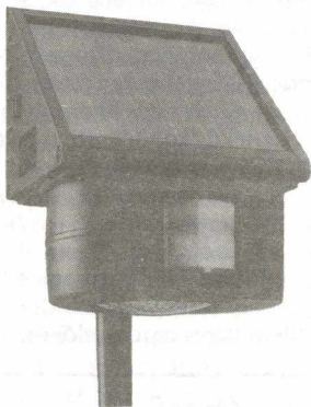
Az ábrán egy kerti lámpa látható, mely egybeépítve tartalmazza a napelemet, az akkut, a lámpát, a közeli-téskapcsolót és a szabályozó elektronikus áramköröket is.
