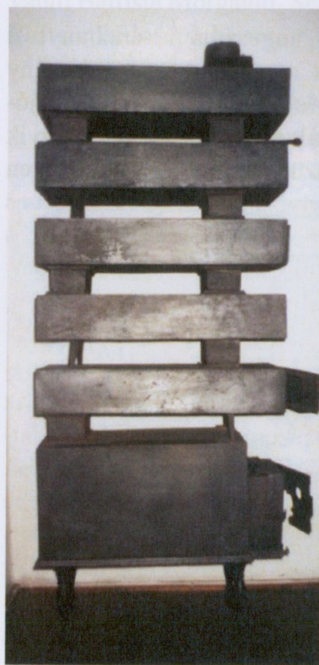
Balra Bolyai Farkas öntöttvaskemencéje Marosvásárhelyen a Bolyai-Múzeumban (Teleki Téka); Jobbra ennek mintájára készült ún. Dániel-cserépkálya
